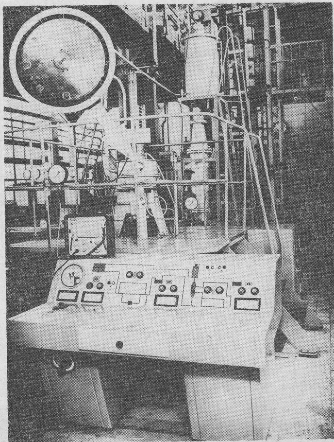
Rys. 1. Ogólny widok stanowiska badawczego (fot. T. Link)
