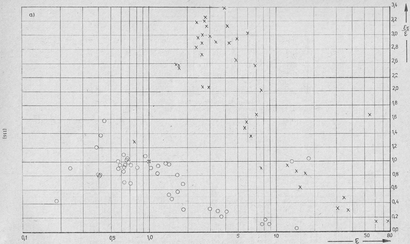
Rys. 13a. Zależność względnego wskaźnika trwałości średniej \varepsilon od wskaźnika względnego \varepsilon_i/\varepsilon odniesionego do stali OH18N9 (kółka) i miedzi M1 (krzyżyki)
