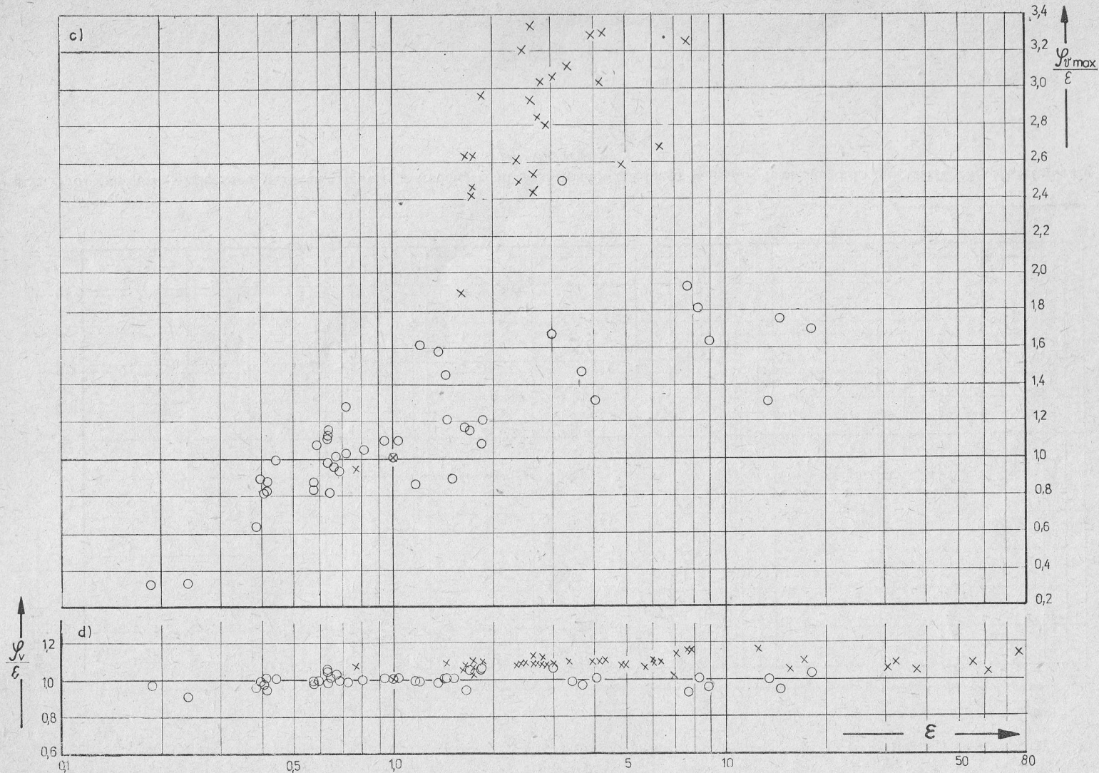
Rys. 13c, d. Zależność względnego wskaźnika trwałości średniej \varepsilon od wskaźników względnych \phi_{vmax}/\varepsilon (c) oraz \phi_v/\varepsilon (d) odniesionych do stali OH18N9 (kółka) i miedzi M1 (krzyżyki)
