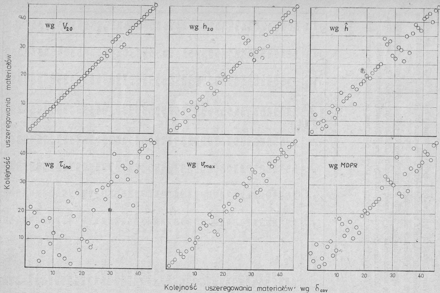
Rys. 12. Względne uszeregowanie badanych materiałów według różnych wskaźników odporności
