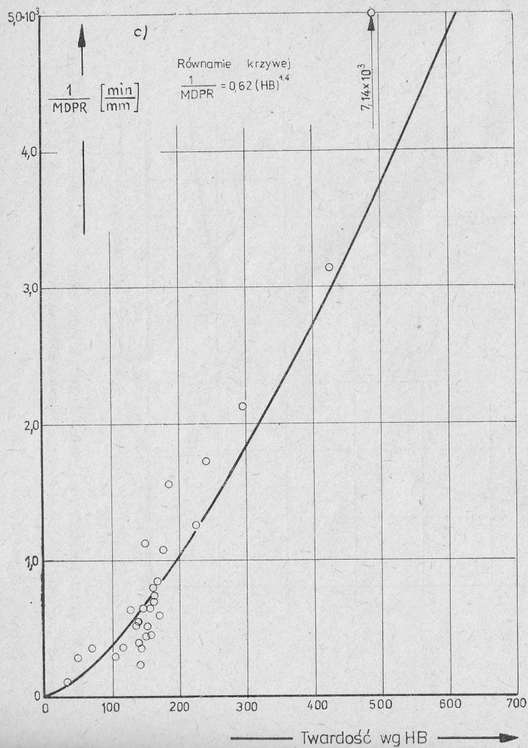
Rys. 14c, d. Związek między twardością (wg HB) stopów żelaza i metali nieżelaznych a ich wskaźnikami odporności 1/MDPR (c) oraz \delta_{cav} (d)
