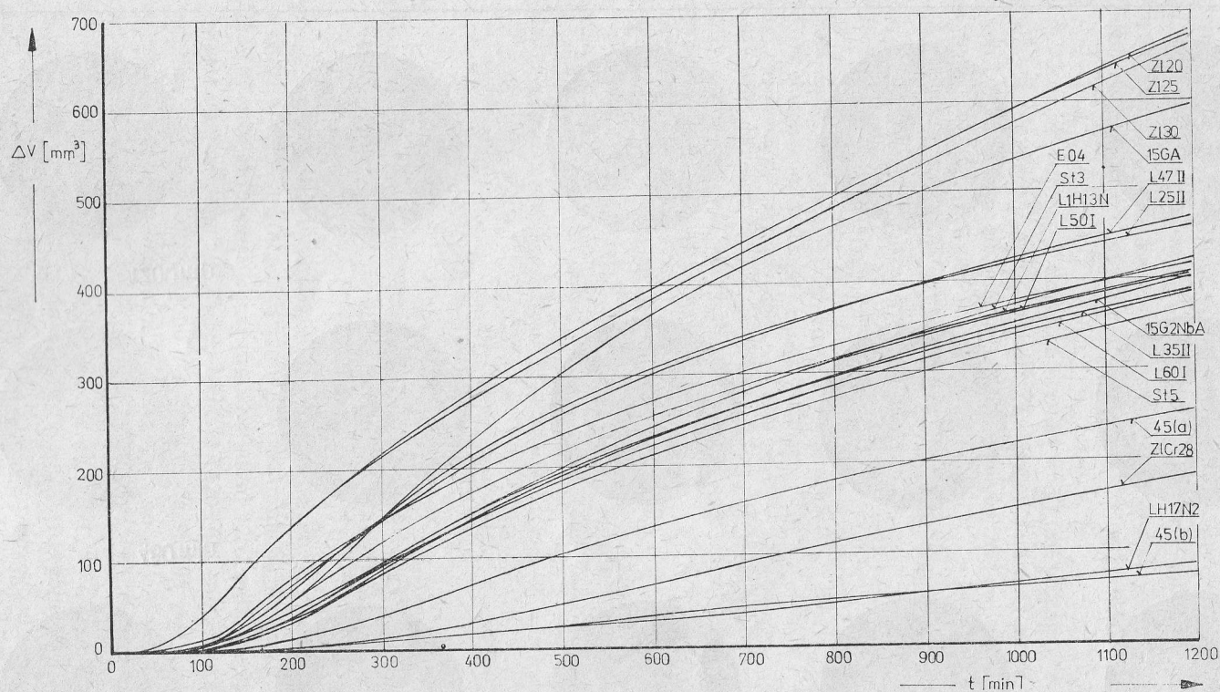
Rys. 5. Wpływ czasu działania kawitacji na ubytek objętościowy próbek z żelaza technicznie czystego i niektórych stopów żelaza
