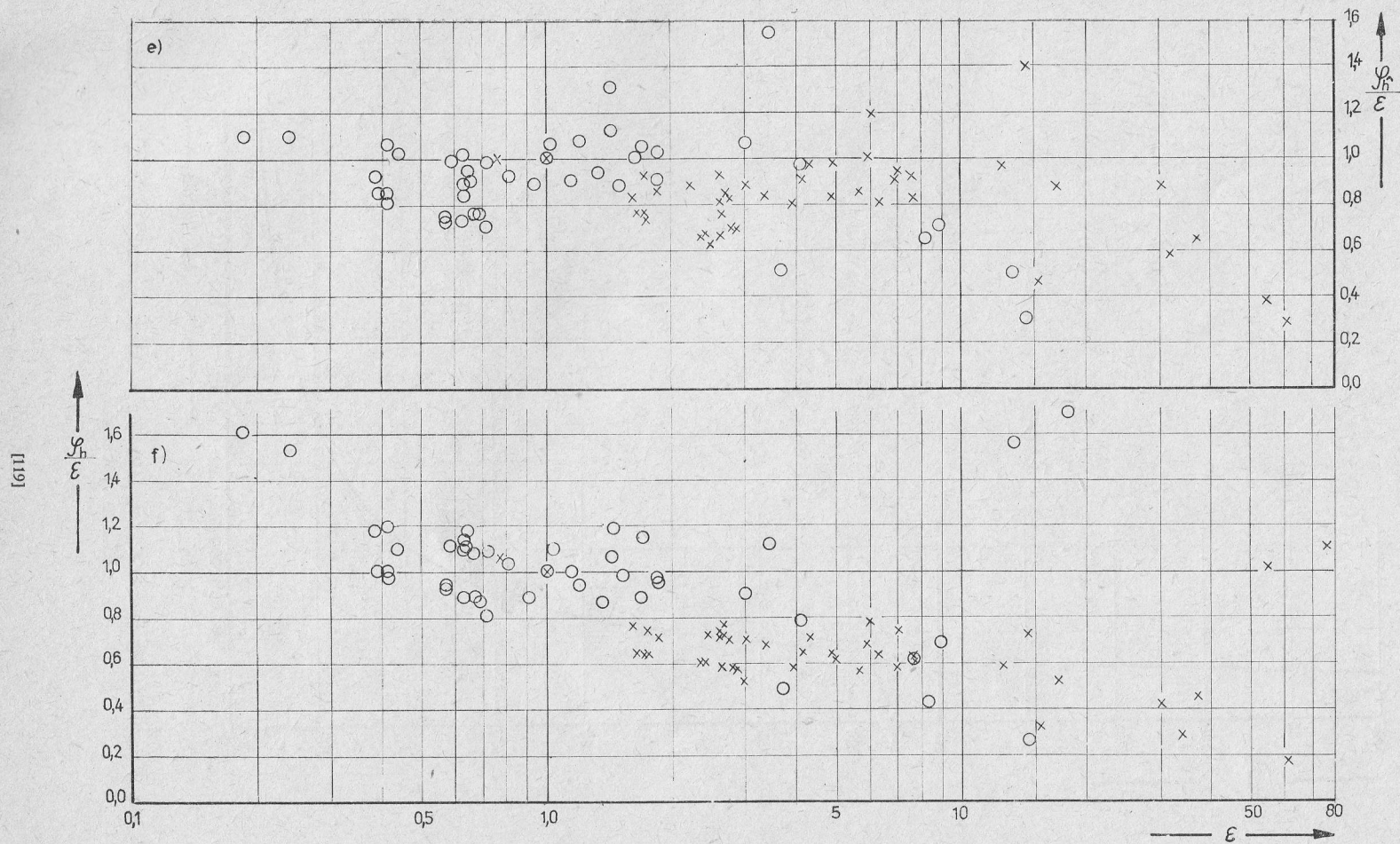
Rys. 13e, f. Zależność względnego wskaźnika trwałości średniej \varepsilon od wskaźników względnych \varphi_h^\Delta/\varepsilon (e) oraz \varphi_h/\varepsilon (f) odniesionych do stali OH18N9 (kółka) i miedzi M1 (krzyżyki)
