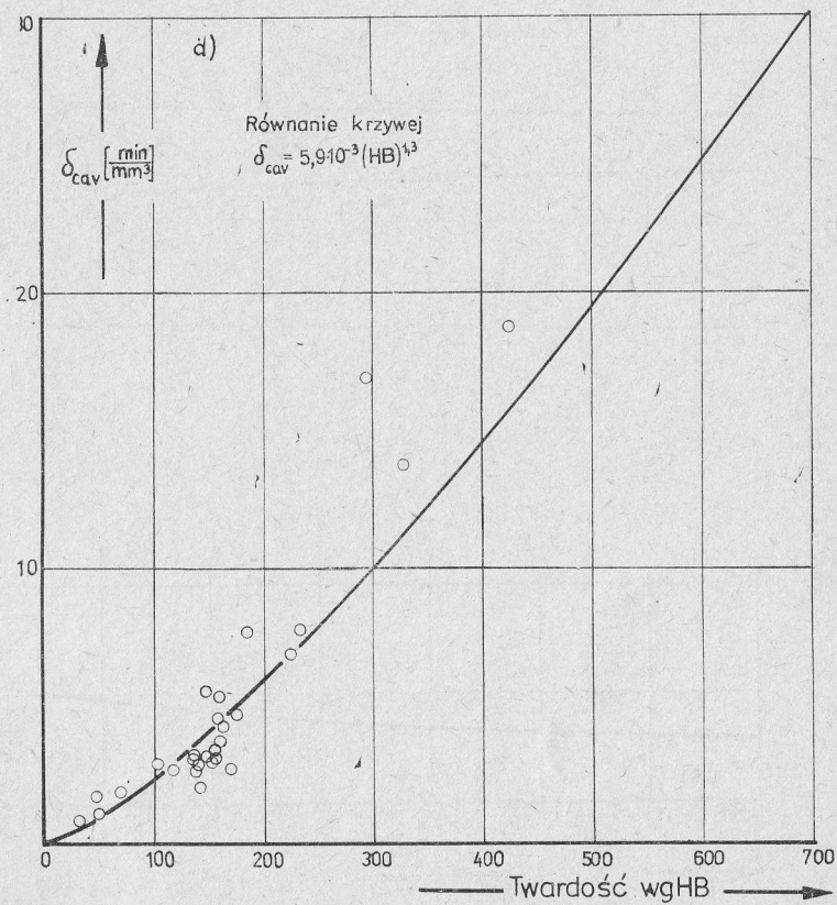
Rys. 14c, d. Związek między twardością (wg HB) stopów żelaza i metali nieżelaznych a ich wskaźnikami odporności 1/MDPR (c) oraz \delta_{cav} (d)
