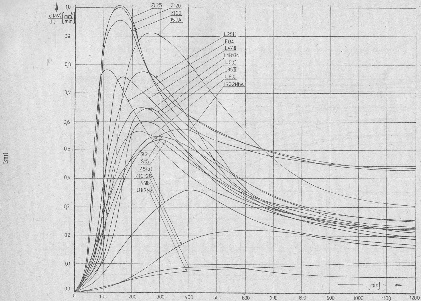
Rys. 8. Zależność szybkości erozji próbek z żelaza technicznie czystego i niektórych stopów żelaza od czasu działania kawitacji
