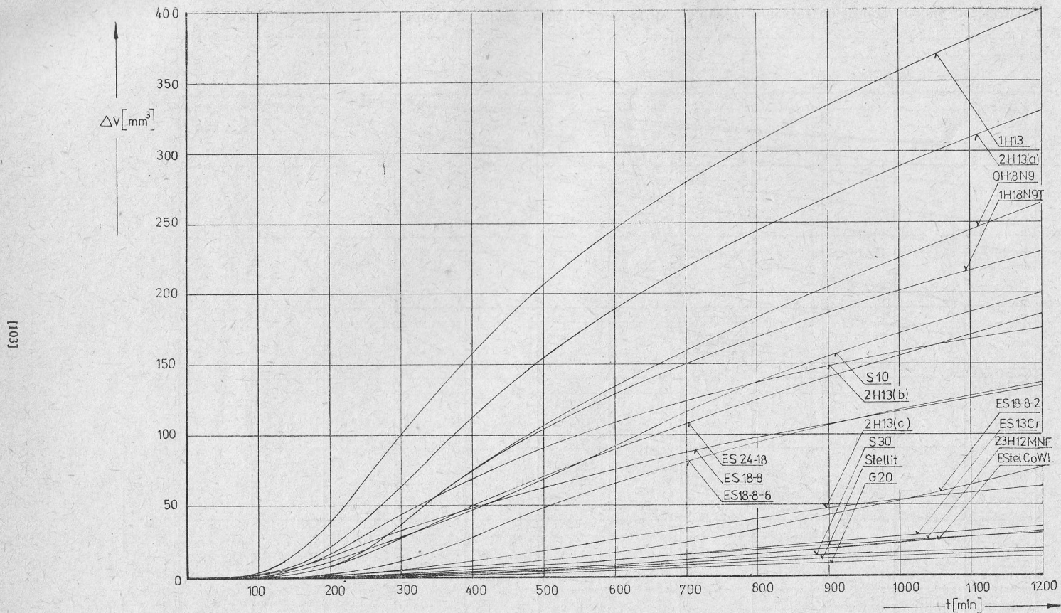
Rys. 6 Wpływ czasu działania kawitacji na ubytek objętościowy próbek ze stopów żelaza i węglków spiekanych
