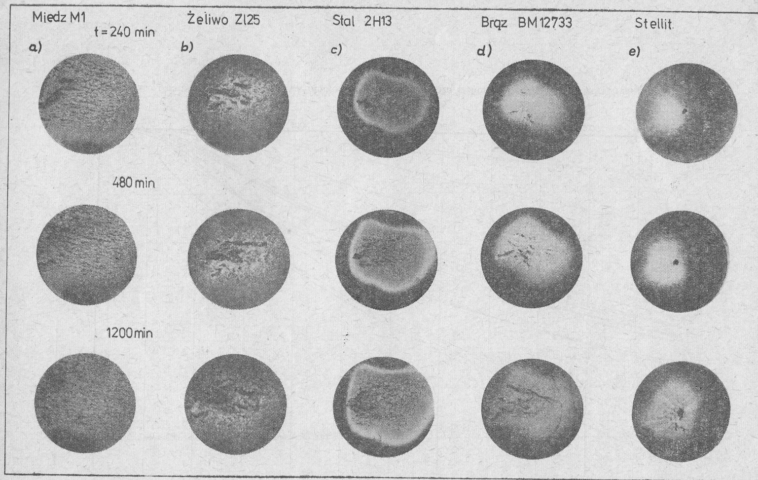
Rys. 4. Topografia powierzchni niektórych próbek po 240, 480 i 1200 min ekspozycji; a) miedź elektrolityczna M1, b) żeliwo ZI25, c) stal nierdzewna 2H13, d) brąz BM12733, e) stellit
