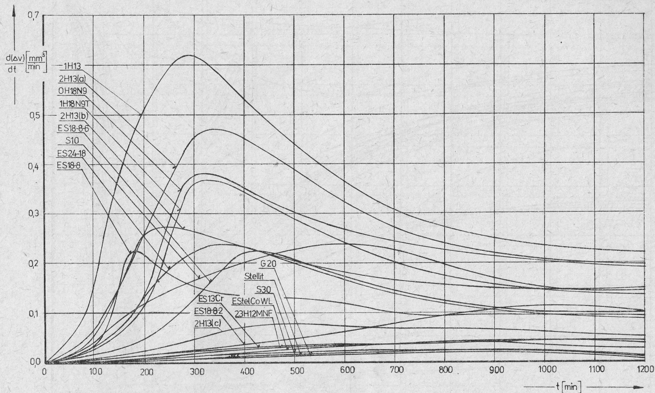
Rys. 9. Zależność szybkości erozji próbek ze stopów żelaza i węglików spiekanych od czasu działania kawitacji
