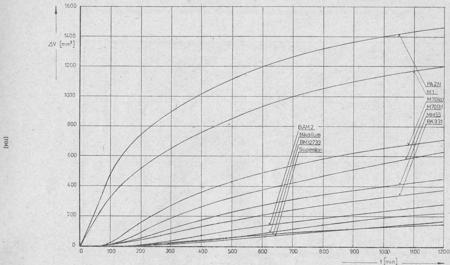
Rys. 7. Wpływ czasu działania kawitacji na ubytek objętościowy próbek z miedzi i niektórych stopów metali nieżelaznych
