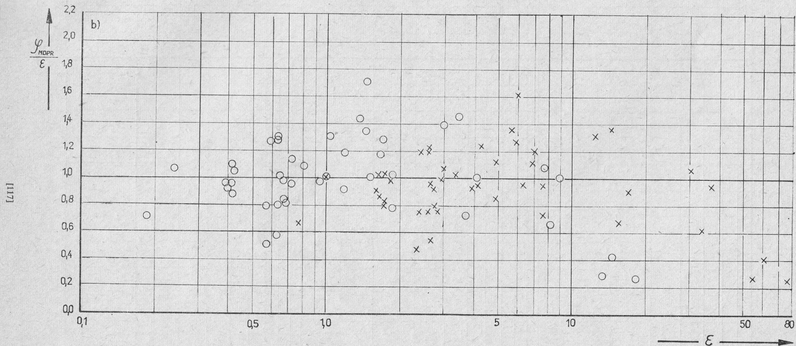
Rys. 13b. Zależność względnego wskaźnika trwałości średniej \varepsilon od wskaźnika względnego \varphi_{MDPR}/\varepsilon odniesionego do stali OH18N9 (kółka) i miedzi M1 (krzyżyki)
