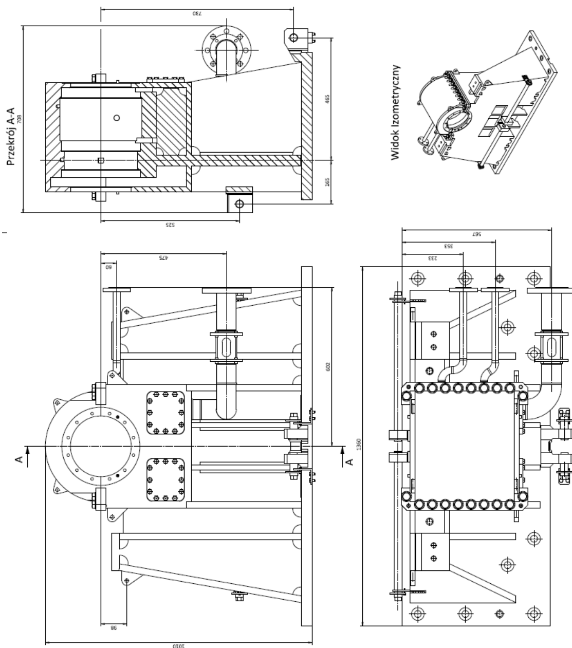
Rys. 4.4 Stojak tylny
