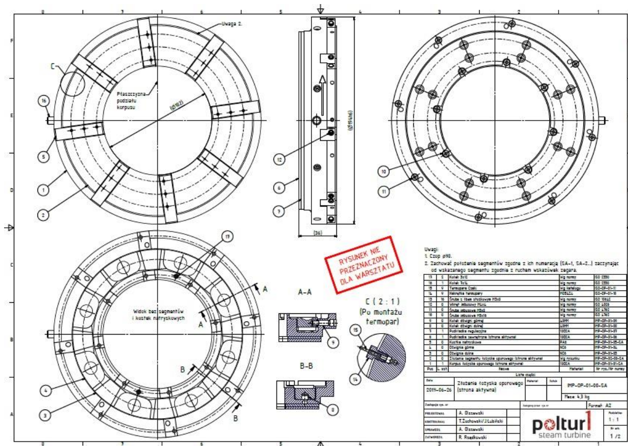
Rys. 4.10 Rysunek złożeniowy łożyska wzdłużnego IMP-OP-01-00-SA
