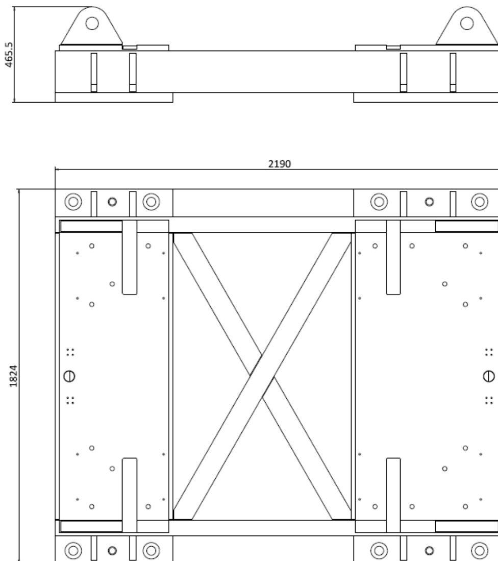
Rys. 4.1. Rama turbiny
