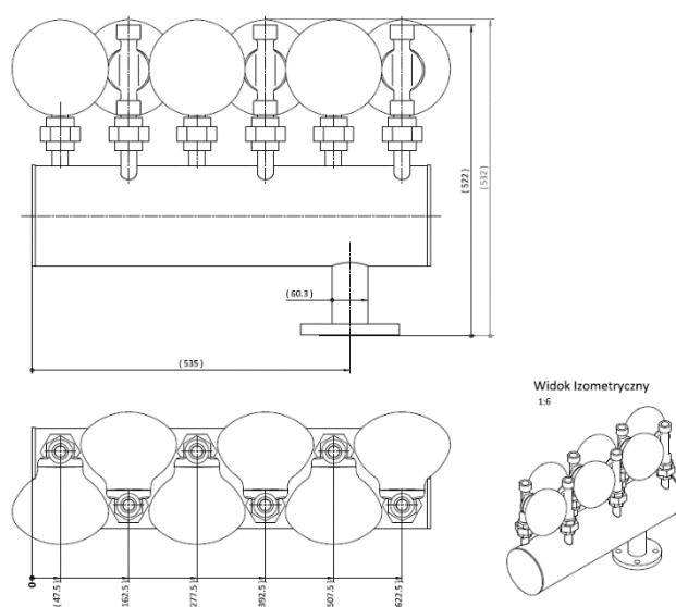
Rys. 4.21 Kolektor skroplin
