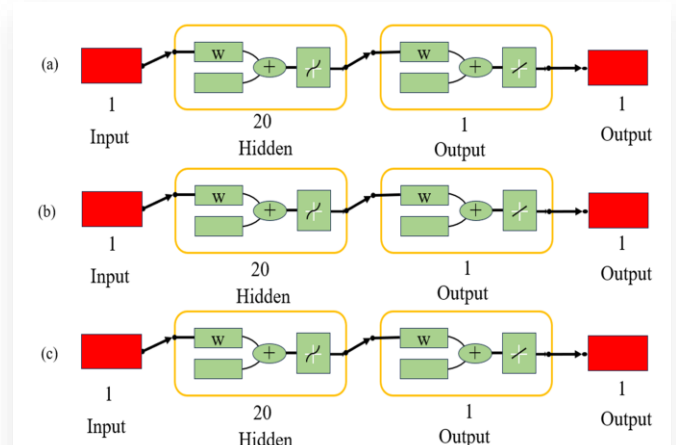
Fig. 20. ANN design.
